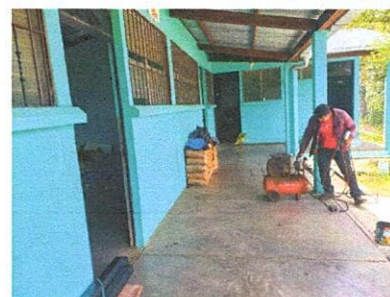
Foto 6: Preparación de la superficie y aplicación de pintura a dos manos, en paredes interiores y exteriores del establecimiento.
